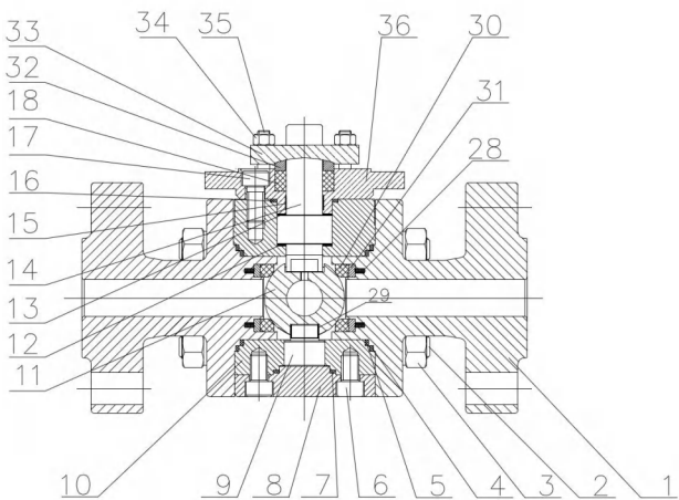
DN65 - DN300 PTFE Packing
