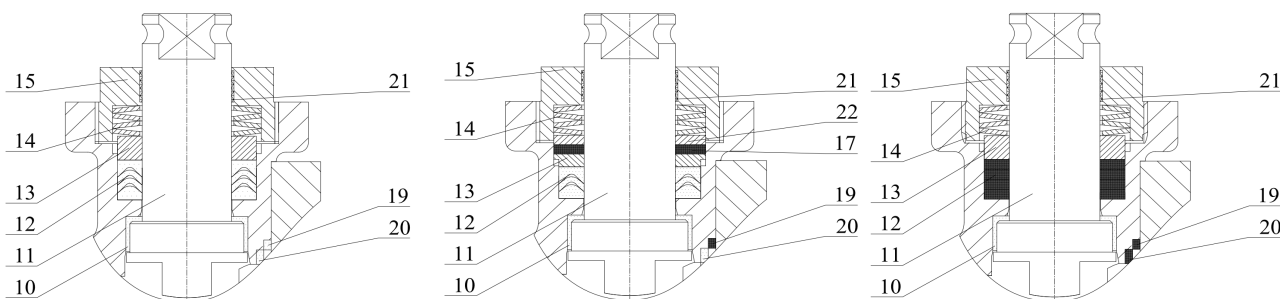
NP(Nut, PTFE)
